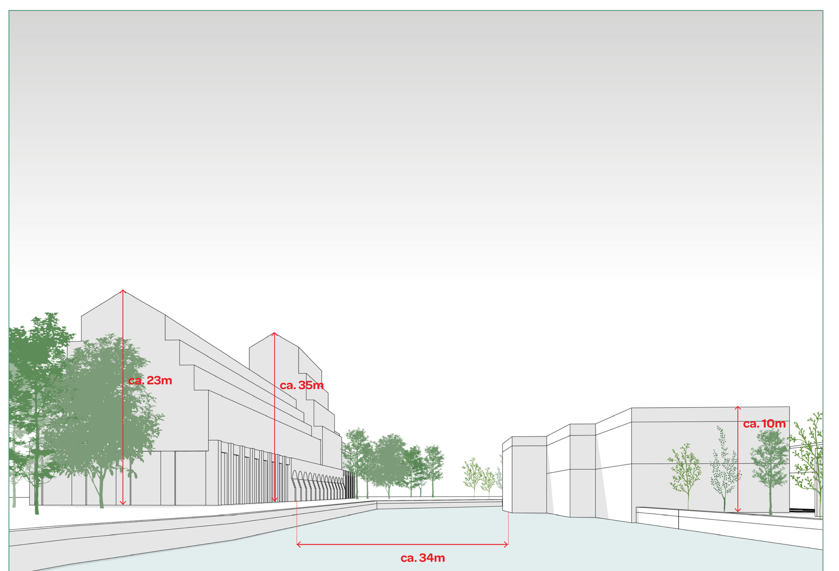
Perspectief waterzijde
